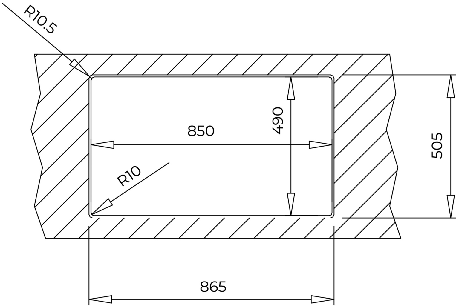
Ausschnitt für flächenbündige Spüle
